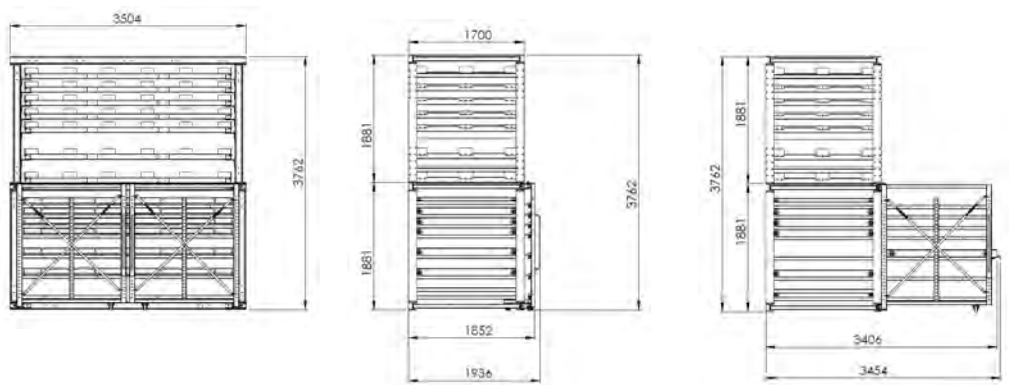
Maßangaben FETZER CUBE Großformat
